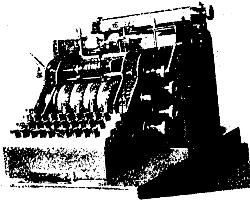
Abb. 2. Chiffriermaschine ohne Verschlus- kappen.
